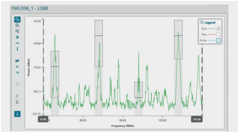
Automatische Störrerkennung mit Hilfe des LS OBSERVER Systems
